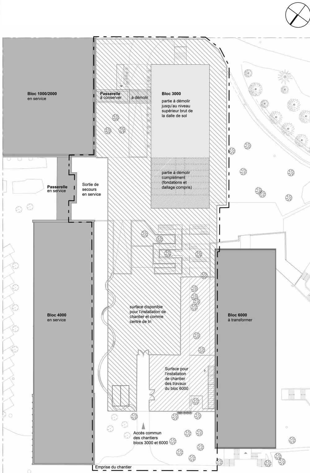
Plan d'installation chantier par Daedalus Engineering.
