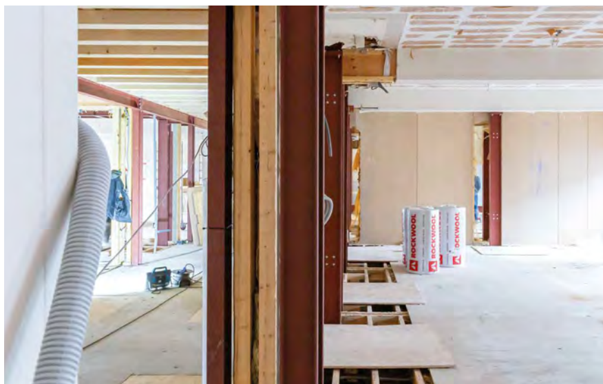
Création des ouvertures dans les murs en ossature bois pour pouvoir réaliser une liaison entre les cadres salle de classe et ceux du couloir.
