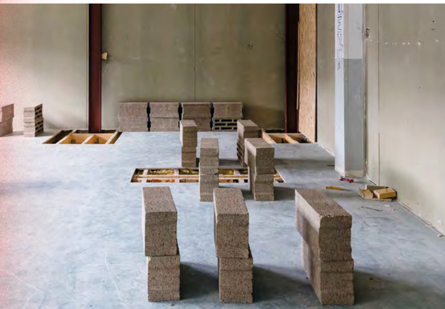
Création des ouvertures dans le plancher du rez-de-chaussée pour les nouvelles fondations.
