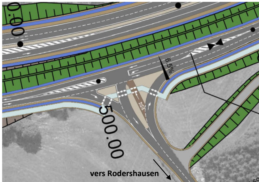
ZOOM 2 Raccord CR342 / Rodershausen
